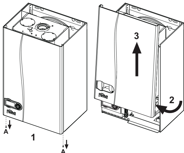
рис. 27 - Снятие кожуха
