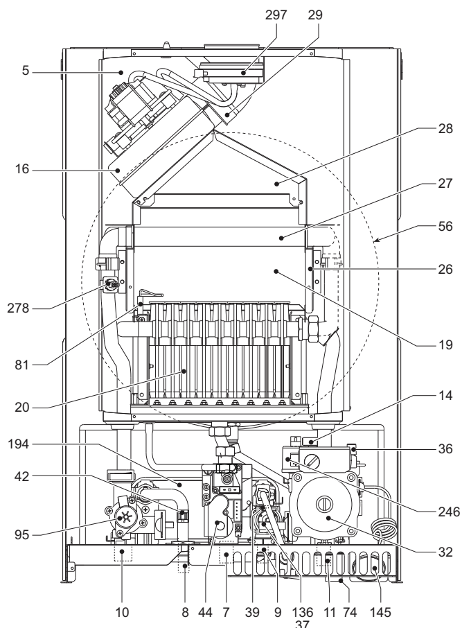
fig. 29 - Vedere generală DIVAtop MICRO LN F 24
