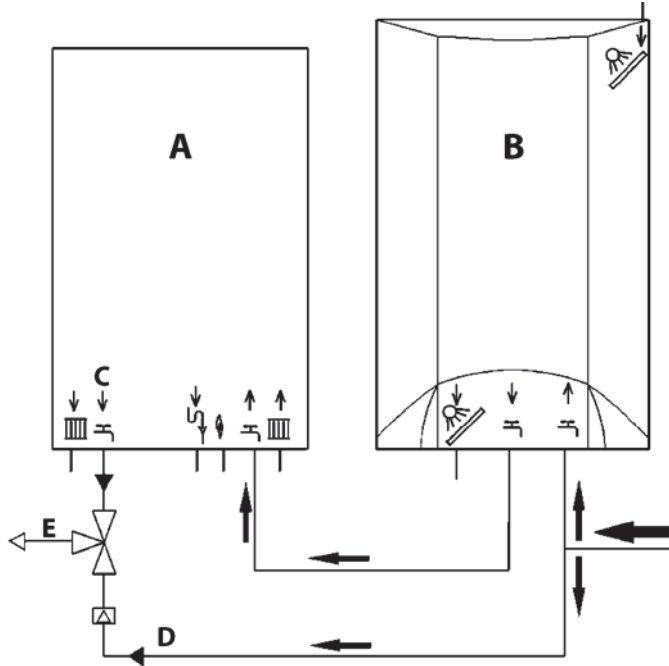
şek. 18 - Güneş enerjisi sistem şeması
