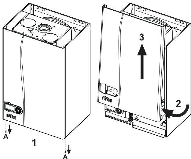
fig. 27 - Deschiderea carcasei
