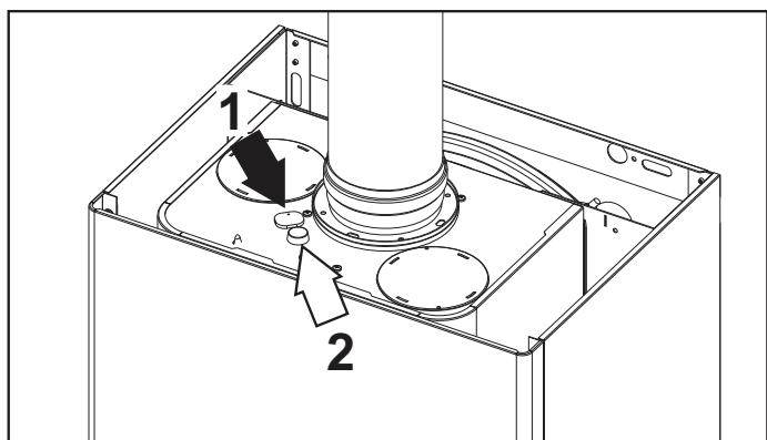
fig. 28 - Analyse des fumées DIVAtop MICRO LN F 24
