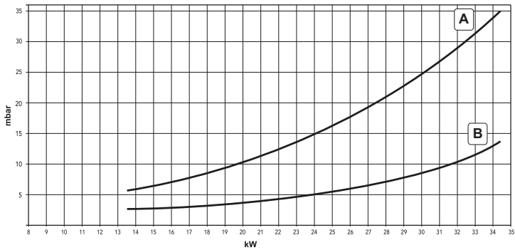
fig. 33 - Diagramă presiune/putere DIVAtop MICRO LN F 32
