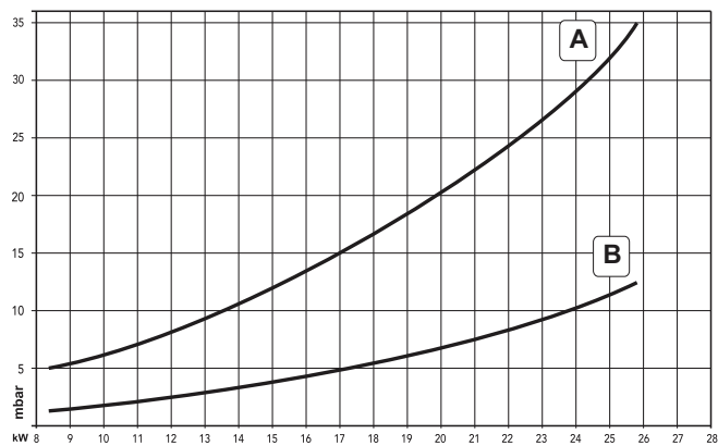
fig. 31 - Diagrama presión / potencia DIVAtop MICRO LN F 24
