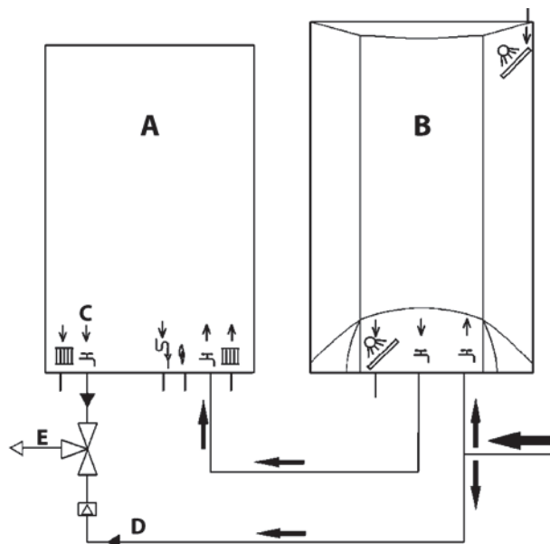
fig. 18 - Schema impianto solare
