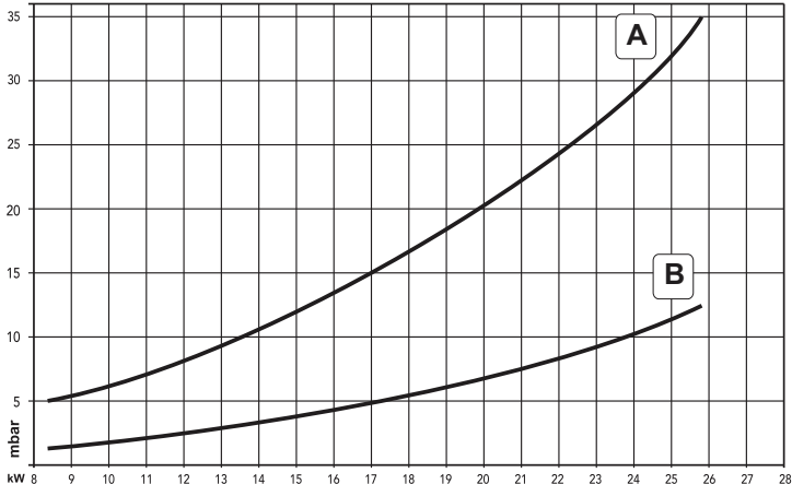
fig. 31 - Diagramă presiune/putere DIVAtop MICRO LN F 24
