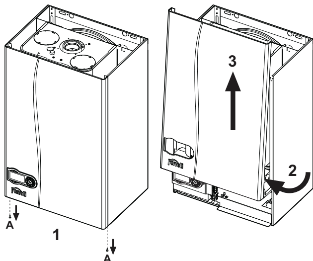
fig. 27 - Démontage de l'habillage
