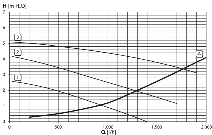
мал. 32 - Утрати напору / тиску циркуляційних насосів DIVAtop MICRO LN F 24
