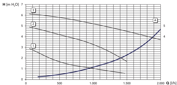
fig. 34 - Pertes de charge / pression circulateurs DIVAtop MICRO LN F 32
