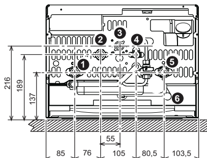
fig. 17 - Attacchi idraulici
