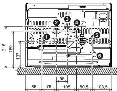
мал. 17 - Гідротехнічні підключення
