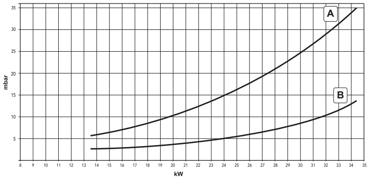
мал. 33 - Діафрагма тиску/потужність DIVAtop MICRO LN F 32
