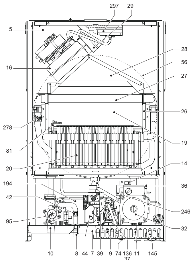
fig. 30 - Vedere generală DIVAtop MICRO LN F 32
