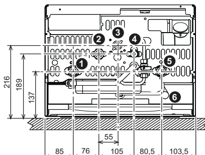
рис. 17 - Гидравлические соединения
