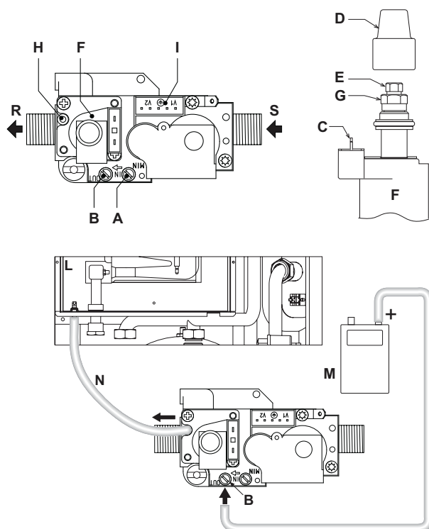
мал. 26 - Газовий клапан
