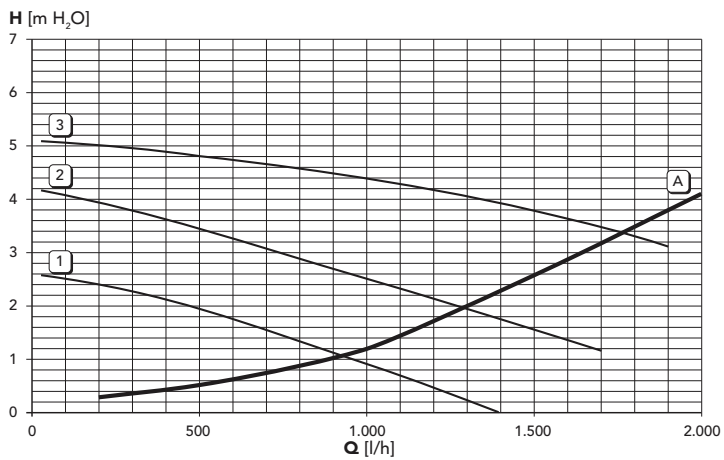
fig. 32 - Pierderi de sarcină / înălțime de pompare pompe de circulație DIVAtop MICRO LN F 24
