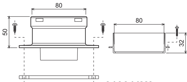
fig. 23 - Accessorio di partenza per condotti separati
