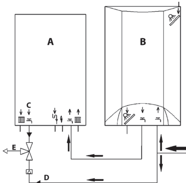
fig. 18 - Schéma installation solaire
