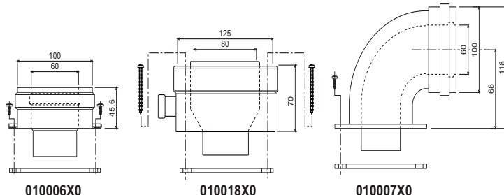
fig. 21 - Accesorii de plecare pentru conducte coaxiale
