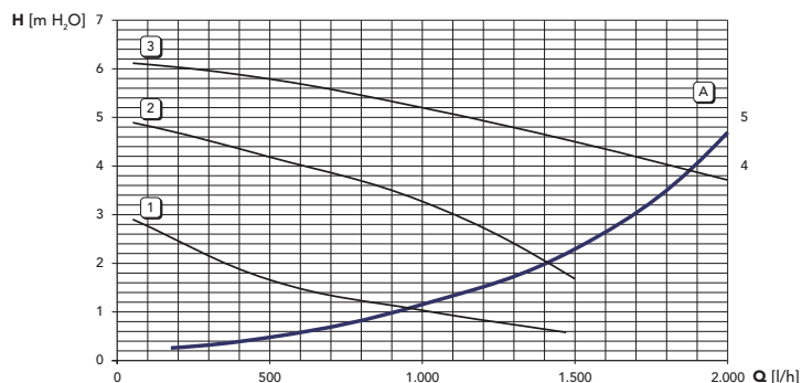
рис. 34 - Потери напора циркуляционных насосов DIVAtop MICRO LN F 32
