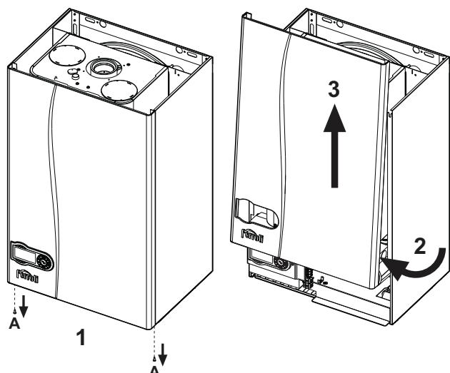
fig. 27 - Apertura mantello
