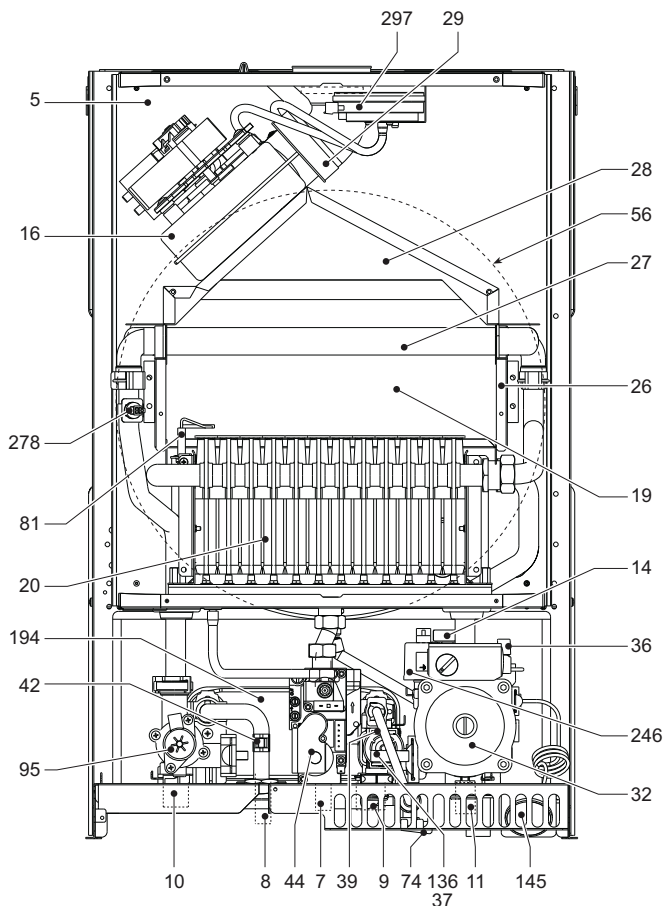
рис. 30 - Общий вид DIVAtop MICRO LN F 32
