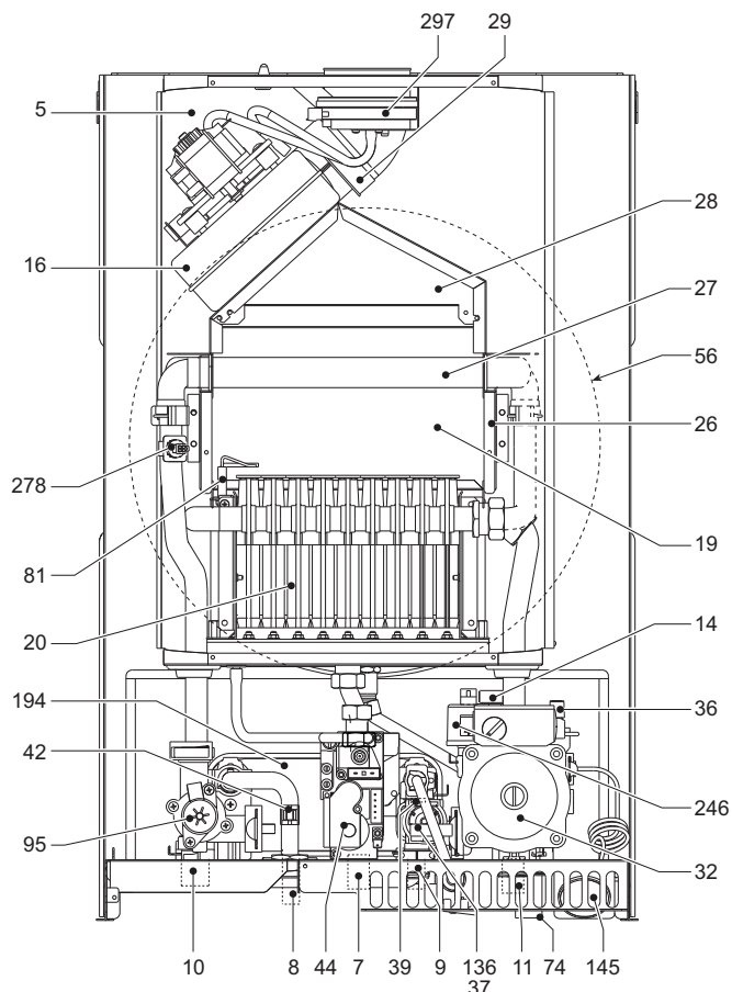
fig. 29 - Vista generale DIVAtop MICRO LN F 24
