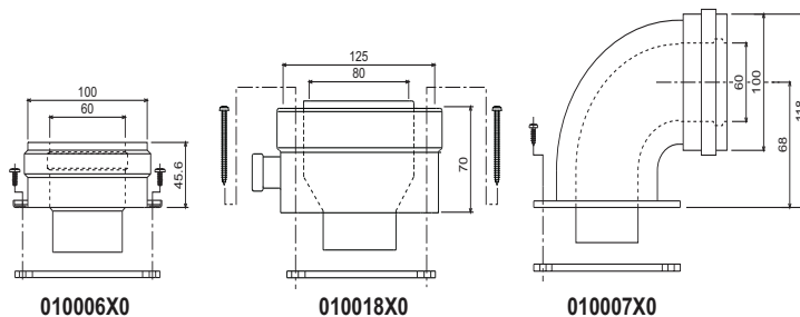
fig. 21 - Accessoires de départ pour conduits coaxiaux
