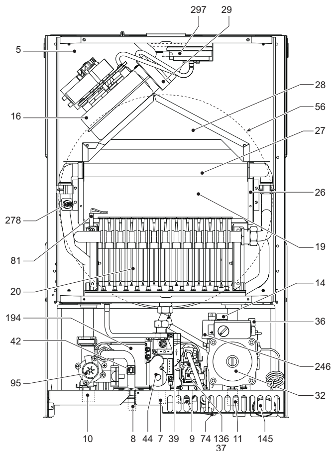
fig. 30 - Vista generale DIVAtop MICRO LN F 32
