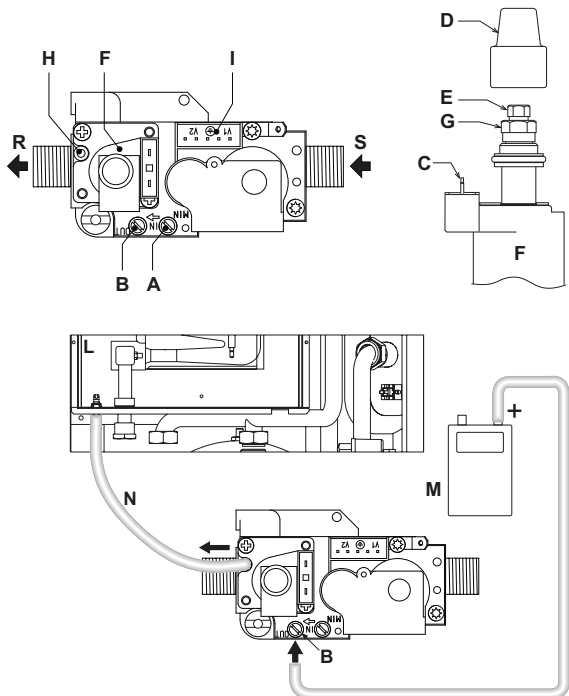
рис. 26 - Газовый клапан
