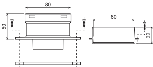
мал. 23 - Початковий елемент для відокремлених трубопроводів
