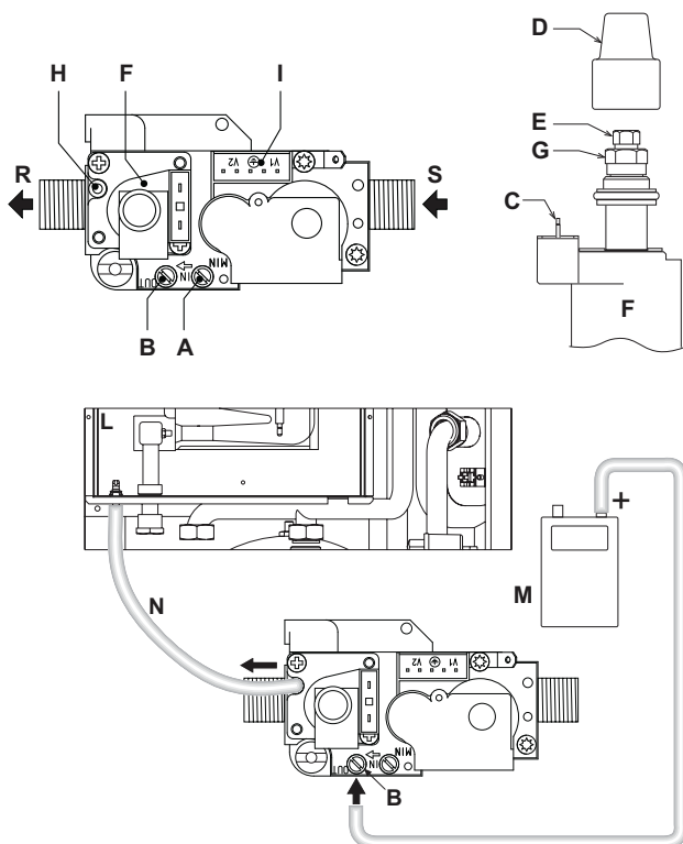
fig. 26 - Válvula de gas
