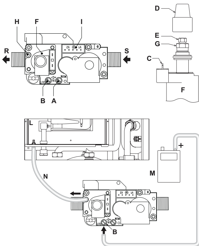
fig. 26 - Valvă de gaz
