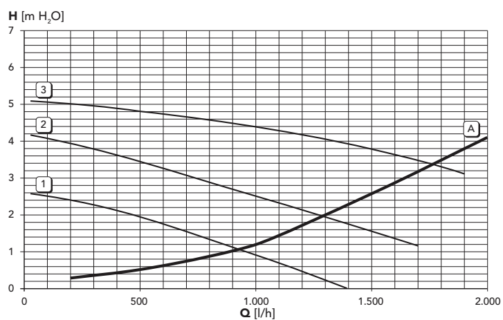
fig. 32 - Pertes de charge / pression circulateurs DIVAtop MICRO LN F 24
