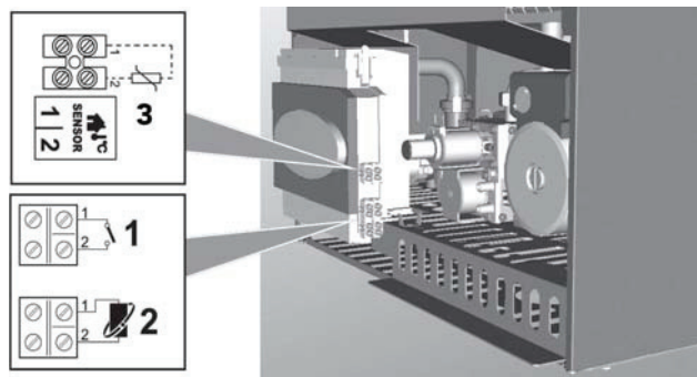
рис. 19 - Доступ к клеммной коробке
