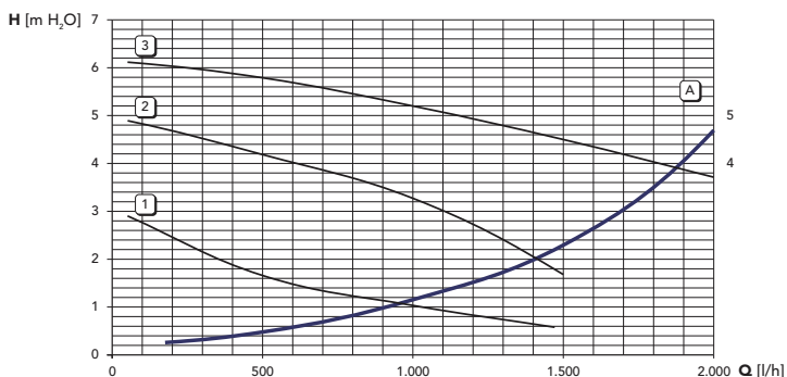
fig. 34 - Pierderi de sarcină / înălțime de pompare pompe de circulație DIVAtop MICRO LN F 32
