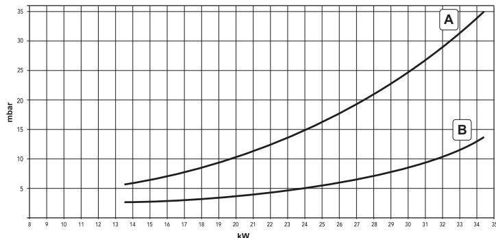
fig. 33 - Diagrama presión / potencia DIVAtop MICRO LN F 32
