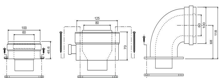
мал. 21 - Початкові елементи для коаксіальних трубопроводів
