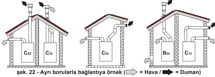
şek. 22 - Ayrı borularla bağlantıya örnek (⇨ = Hava / ⇨ = Duman)
