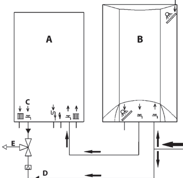
fig. 18 - Schemă instalație solară
