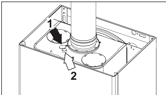
мал. 28 - Аналіз відпрацьованих газів DIVAtop MICRO LN F 24
