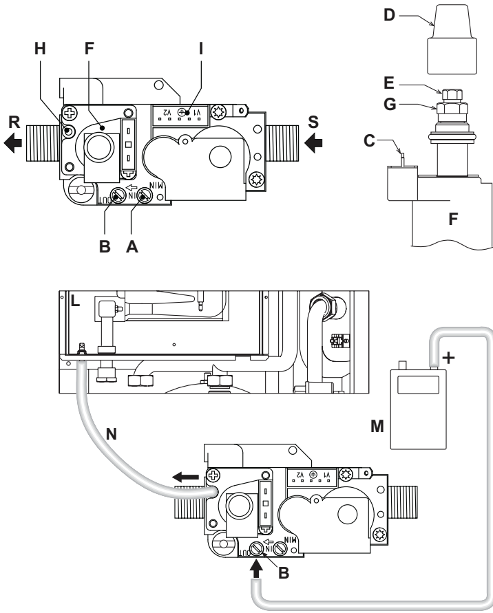
şek. 26 - Gaz valfi
