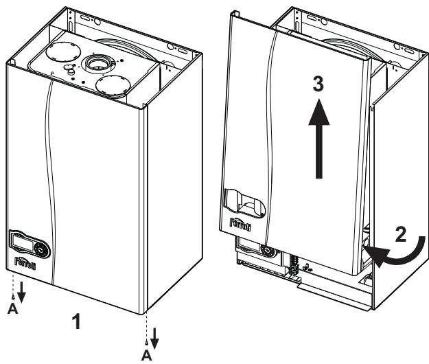
мал. 27 - Зняття кожуха
