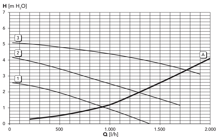
fig. 32 - Pérdidas de carga / carga hidrostática de las bombas de circulación DIVAtop MICRO LN F 24
