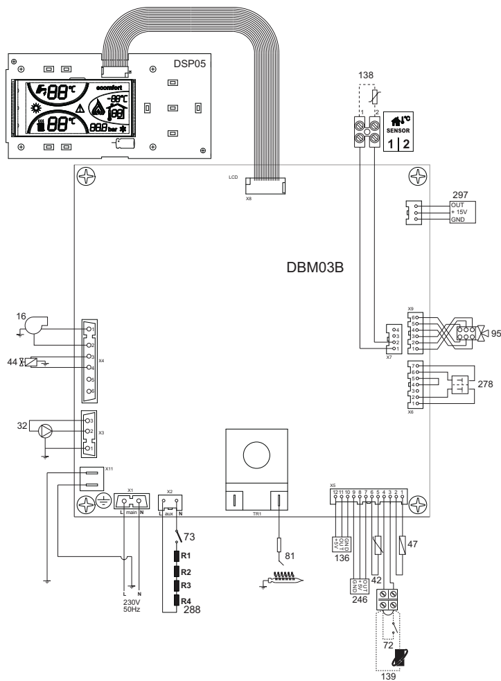
мал. 35 - Електрична схема
