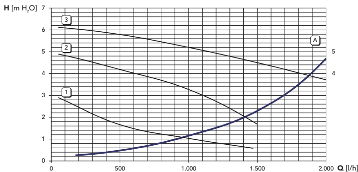
мал. 34 - Утрати напору / тиску циркуляційних насосів DIVAtop MICRO LN F 32
