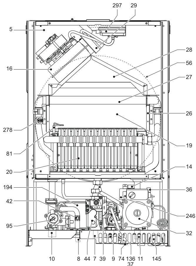
мал. 30 - Загальний вигляд DIVAtop MICRO LN F 32
