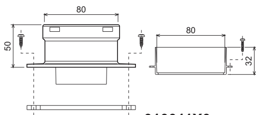
рис. 23 - Соединительный элемент для раздельных труб
