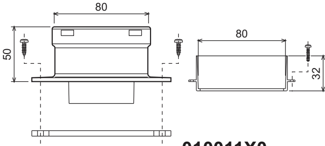
şek. 23 - Ayrı kanallar için çıkış aksesuarları
