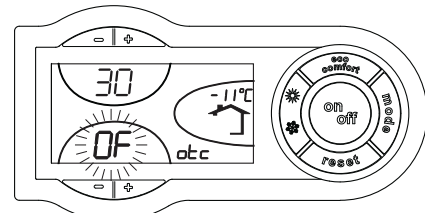
fig. 13 - Desplazamiento paralelo de las curvas
