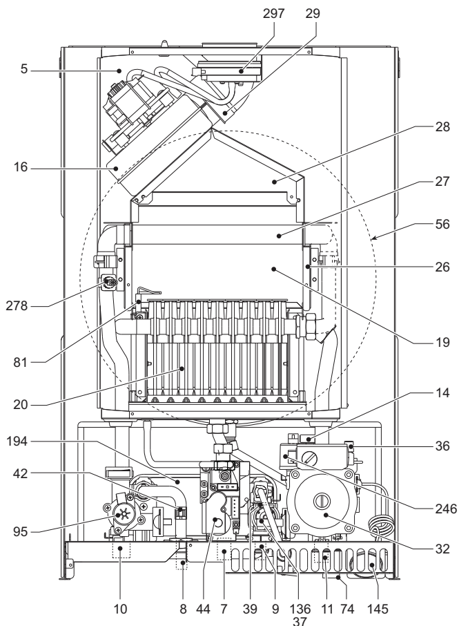
fig. 29 - Vue générale DIVAtop MICRO LN F 24
