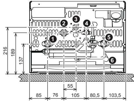
şek. 17 - Su bağlantıları
