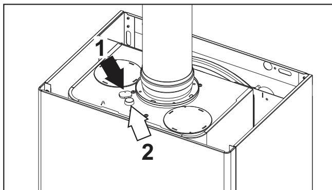
рис. 28 - Анализ продуктов сгорания DIVAtop MICRO LN F 24
