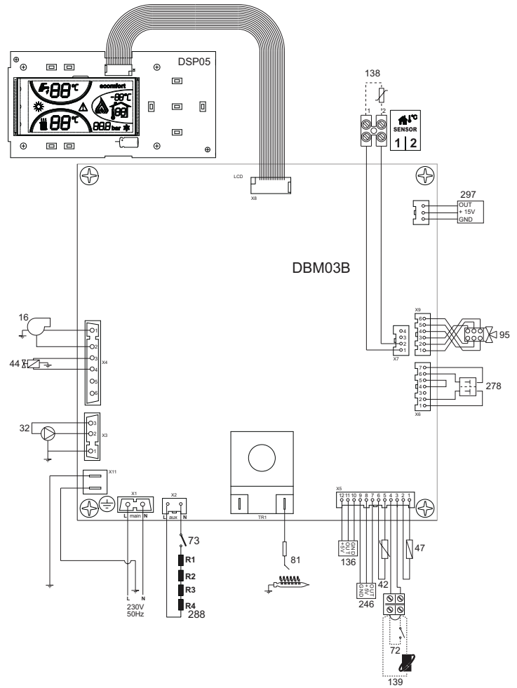
fig. 35 - Schemă electrică
