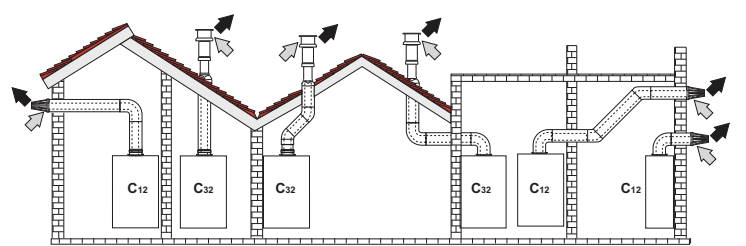
şek. 20 - Koaksiyal borularla bağlantıya örnek (Hava = Hava / Duman = Duman)
