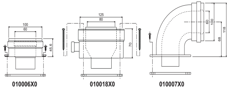
şek. 21 - Koaksiyal kanallar için çıkış aksesuarları
