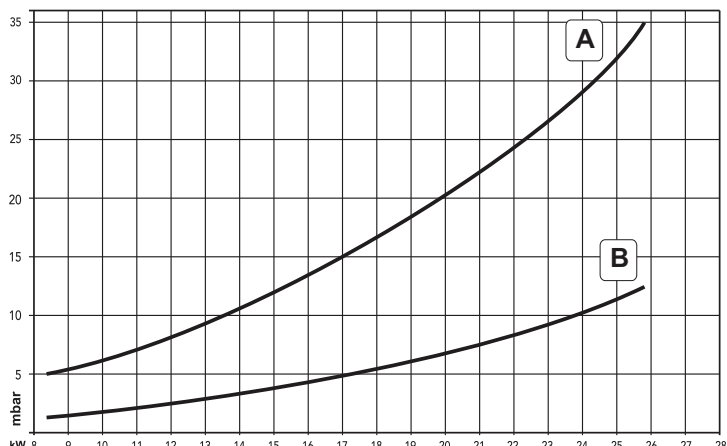
fig. 31 - Diagramma pressione/potenza DIVAtop MICRO LN F 24
