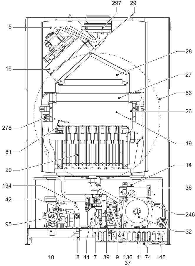
şek. 29 - Genel görünüm DIVAtop MICRO LN F 24
