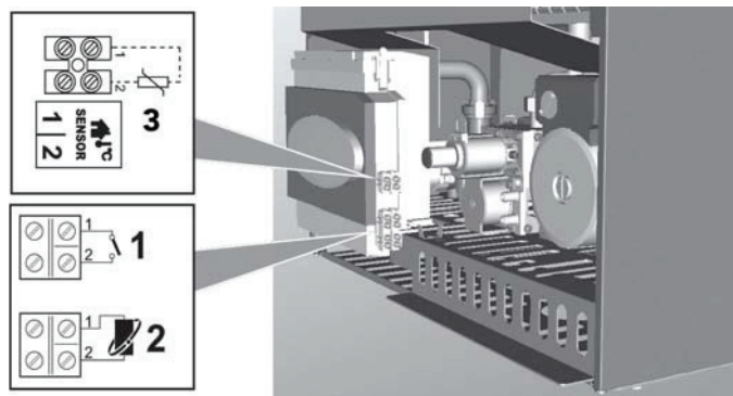
fig. 19 - Accès au bornier
