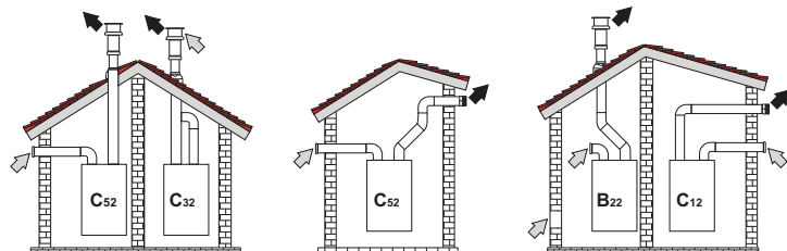
fig. 22 - Exemples de raccords avec conduits séparés (⇨ = Air / ⇨ = Fumées)
