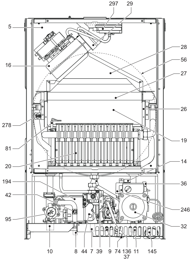
şek. 30 - Genel görünüm DIVAtop MICRO LN F 32
