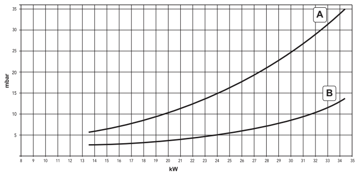
fig. 33 - Diagrammes pression - puissance DIVAtop MICRO LN F 32
