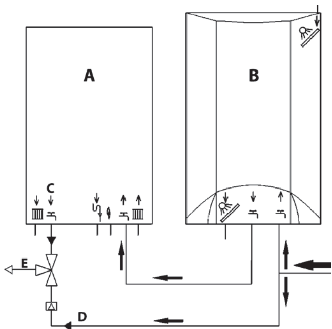
fig. 18 - Esquema de instalación solar
