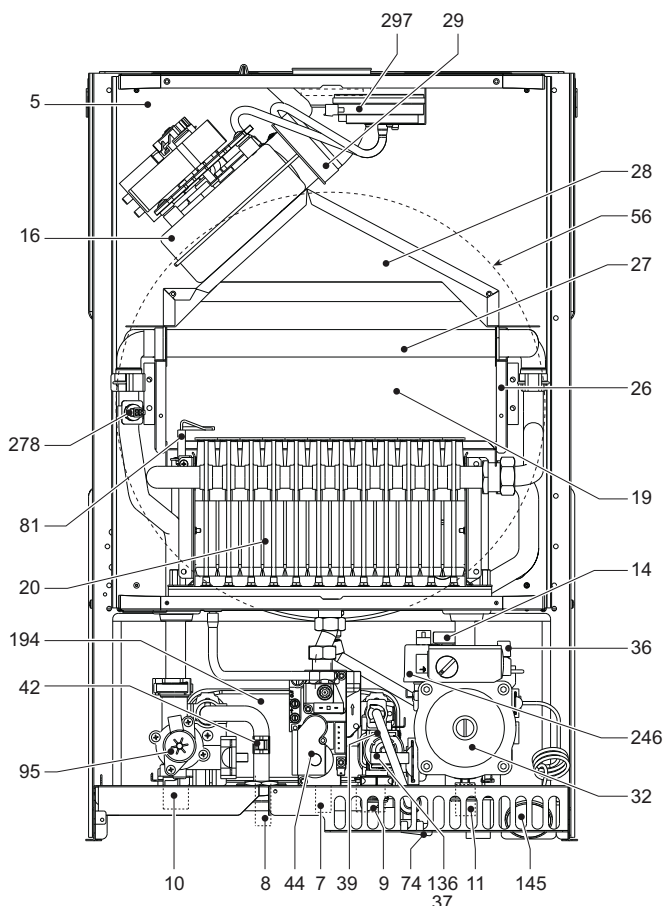
fig. 30 - Vue générale DIVAtop MICRO LN F 32
