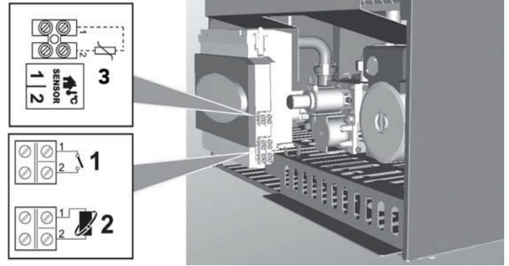
şek. 19 - Elektrik terminaline erişim
