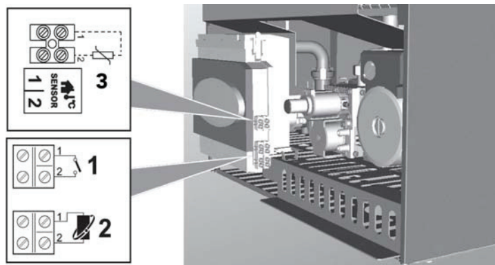
fig. 19 - Accesso alla morsetteria
