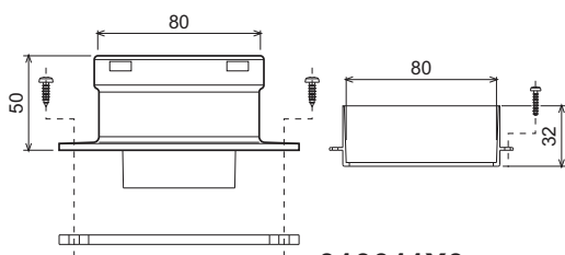
fig. 23 - Accesorio inicial para conductos separados
