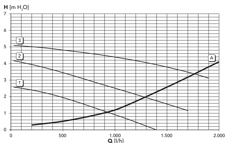
рис. 32 - Потери напора циркуляционных насосов DIVAtop MICRO LN F 24
