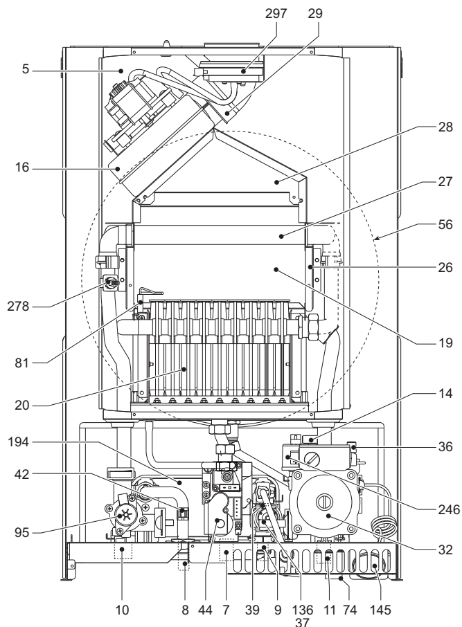
мал. 29 - Загальний вигляд DIVAtop MICRO LN F 24
