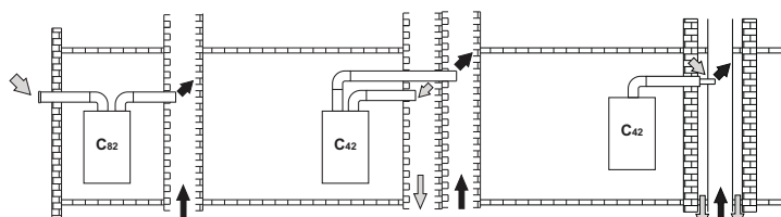
fig. 24 - Exemples de raccords à l'aide de tuyaux coaxiaux (⇨ = Air / ⇨ = Fumées)
