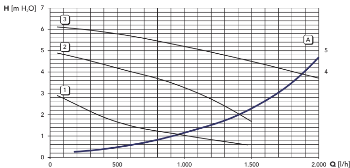
fig. 34 - Pérdidas de carga / carga hidrostática de las bombas de circulación DIVAtop MICRO LN F 32
