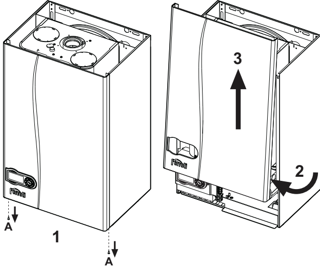
şek. 27 - Muhafazanın/kasanın açılması
