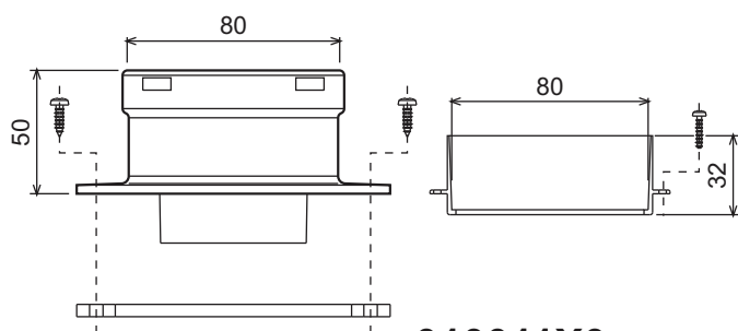
fig. 23 - Accessoire de départ pour conduits séparés
