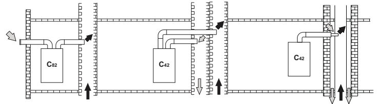
şek. 24 - Duman kanalına bağlantı örneği (⇨ = Hava / ⇨ = Duman)
