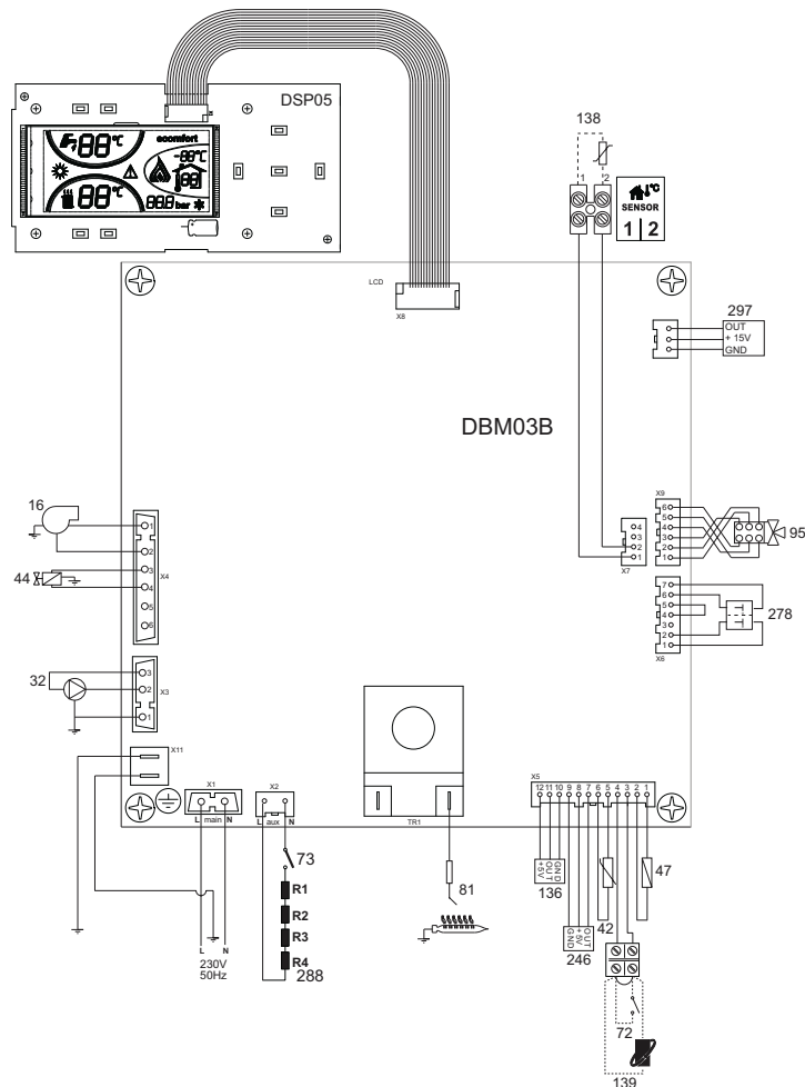
fig. 35 - Esquema eléctrico
