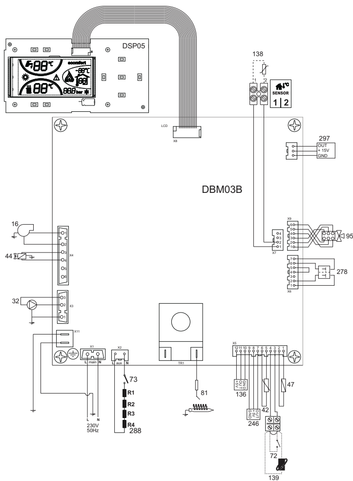
fig. 35 - Schema elettrico
