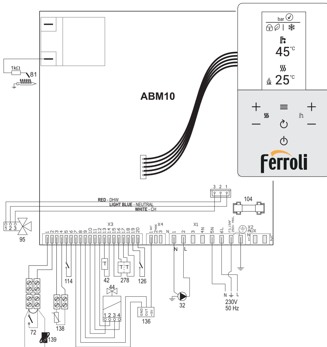
мал. 39- Електрична схема
