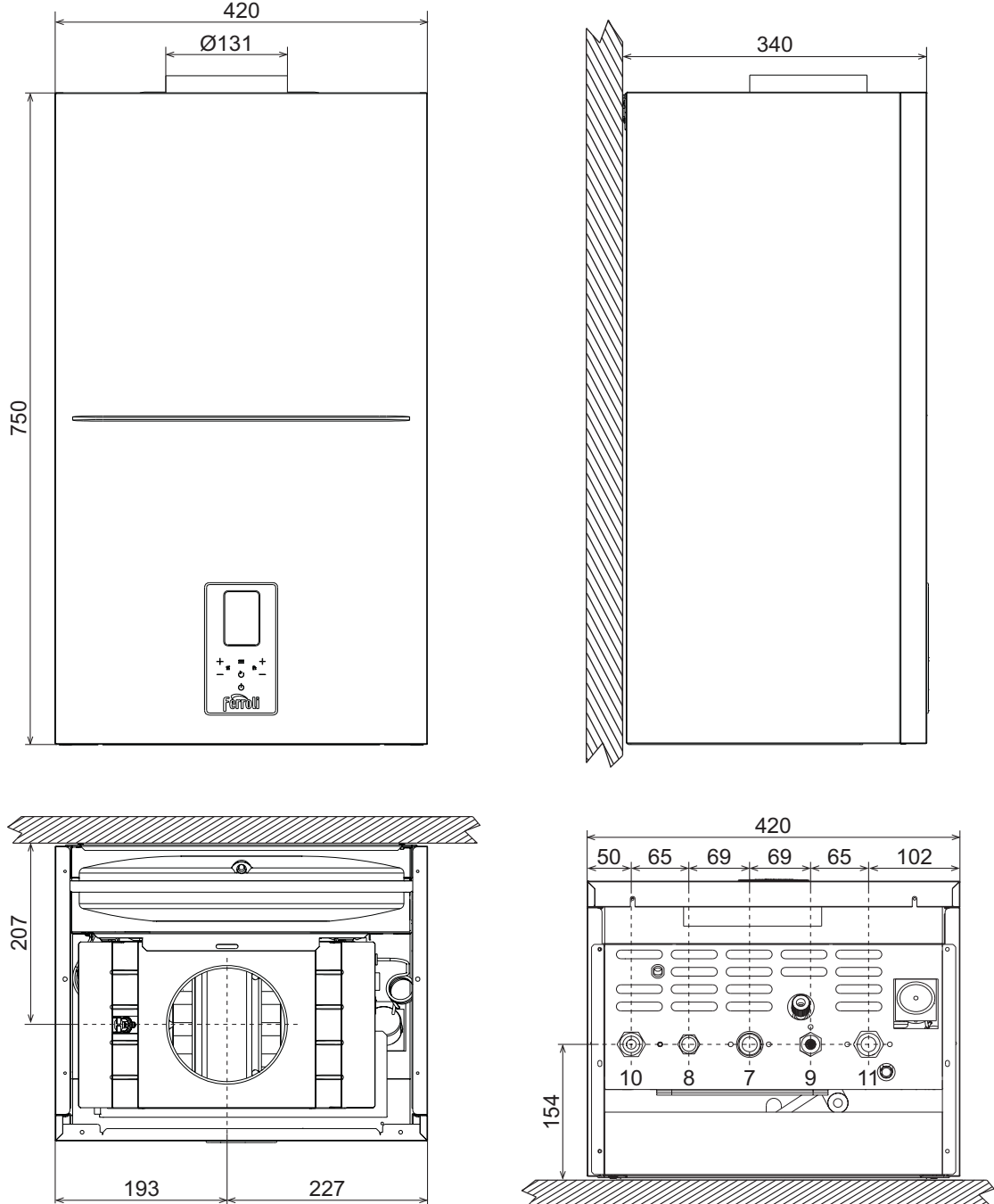
شكل 33 - أبعاد ووصلات الموديل DIVATOP D C24
