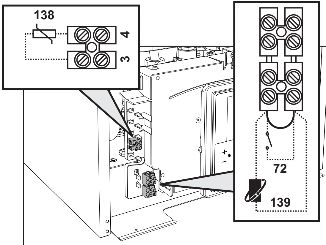
სურ. 25 - ტერმინალურ ბლოკზე წვდომა
