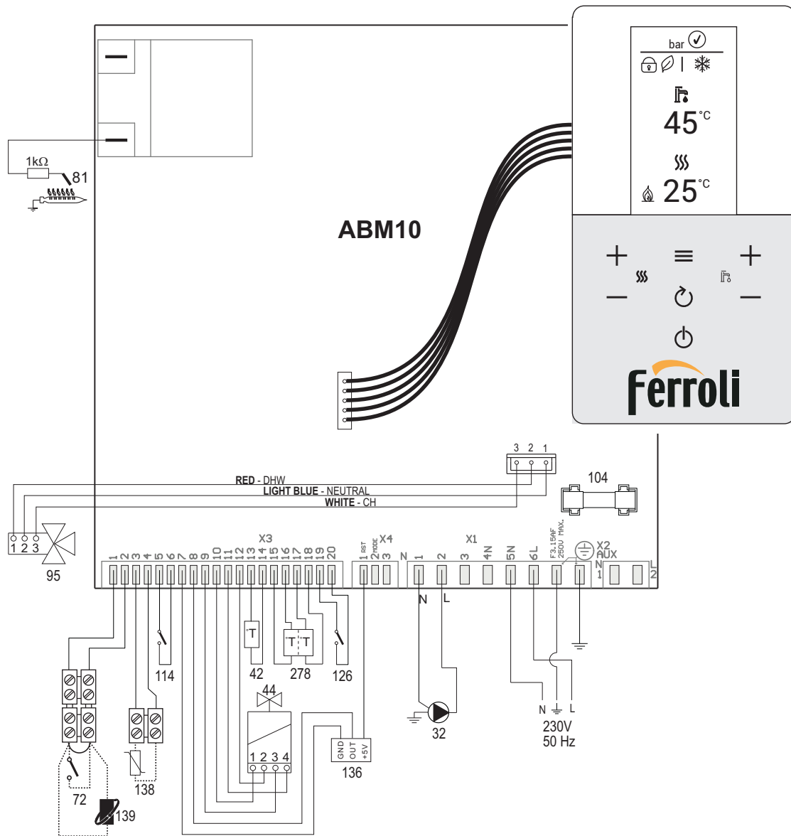
рис. 39- Электрическая схема
