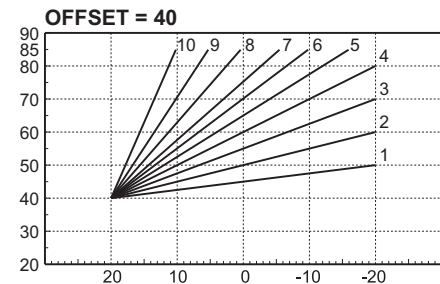
fig. 23- Exemple de déplacement parallèle des courbes de compensation
