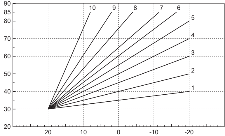
شكل 22 - منحنيات التعويض
