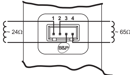
Slika 30- Priključak gasnog ventila
