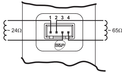
мал. 30 - Підключення газового клапану
