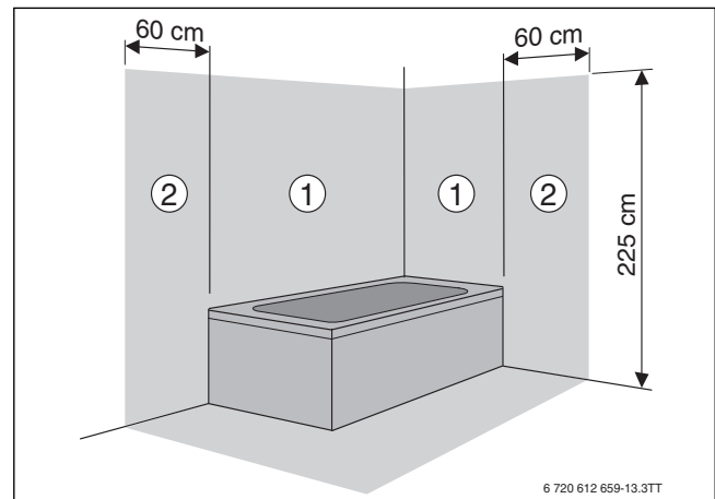
Fig. 26 Áreas de protección
