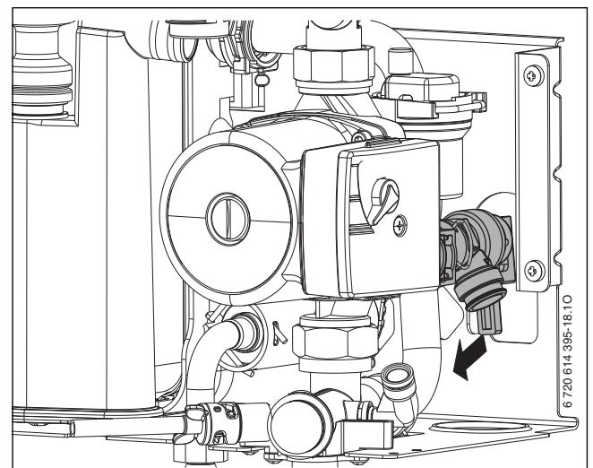
Fig. 56 Válvula de seguridad de la calefacción
